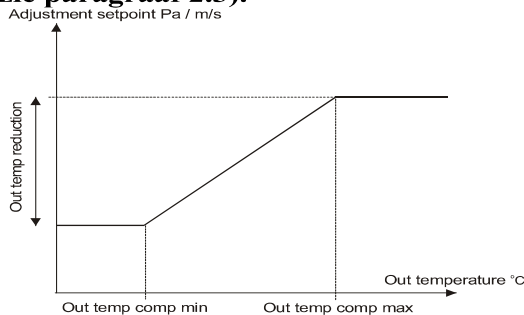
Figuur 2: Buitentemperatuur compensatie.
