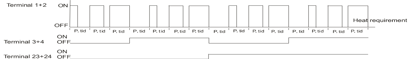
Figuur 1: Puls uitgang sequentie
